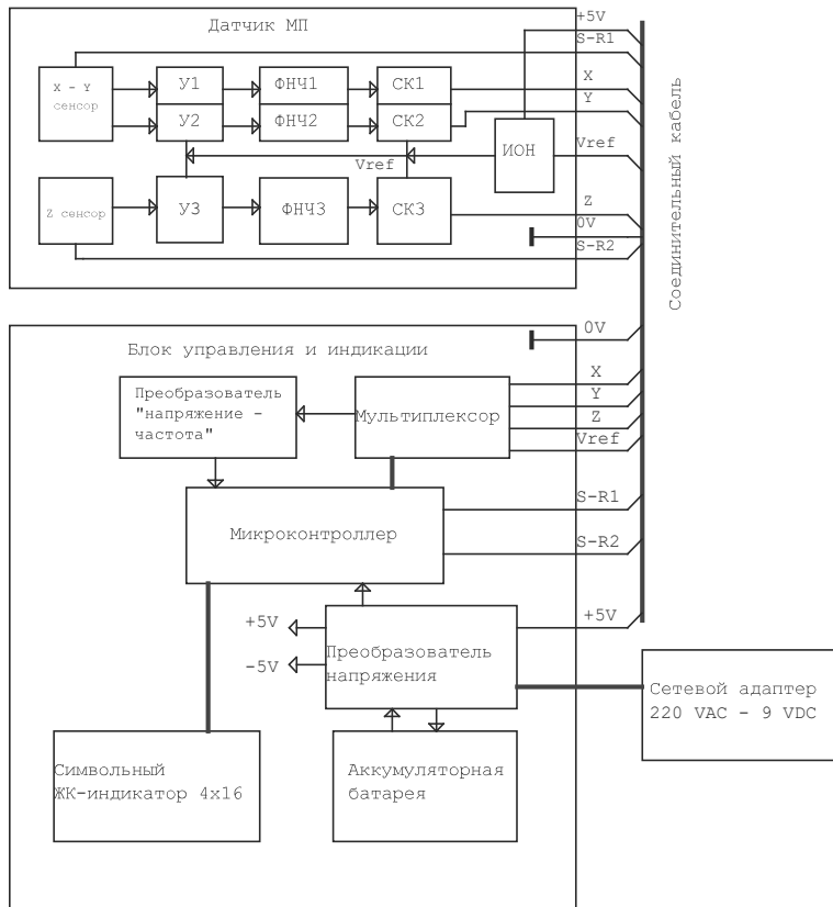
Рисунок 2. Функциональная схема измерителя.
