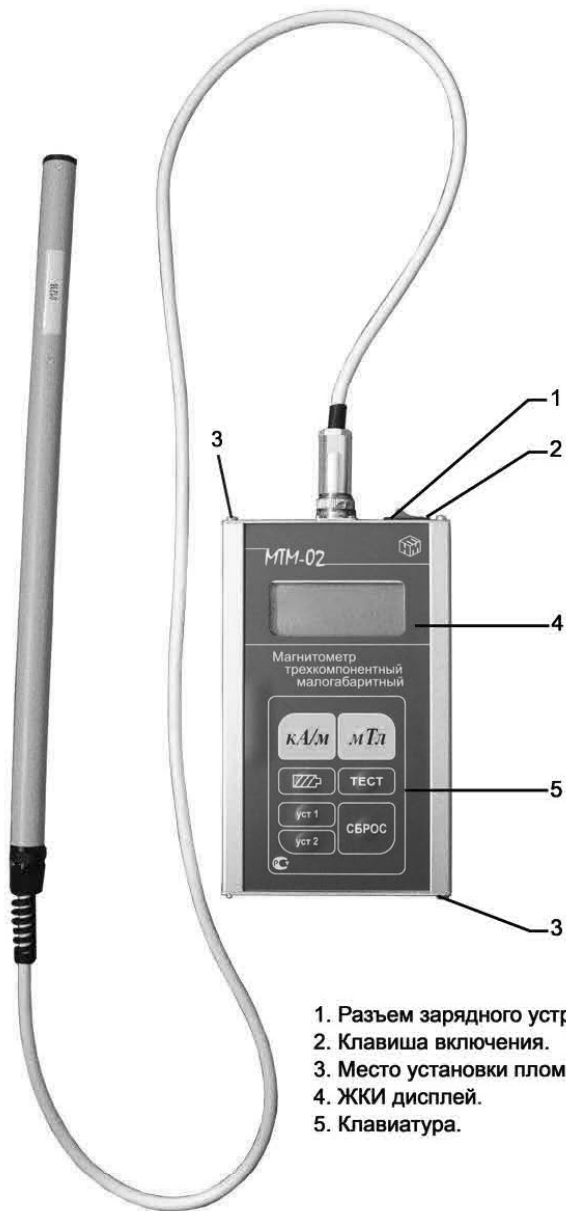
Рисунок 1. Внешний вид измерителя.
