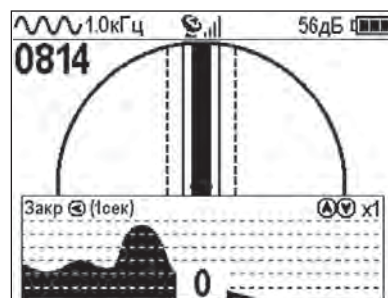
Рис.А.4 КЗ-двухфазное
